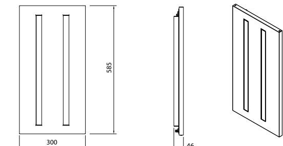
30x60 Sasled Mini Surface Mounted (2 Bar) Luminaire
