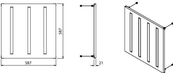
60x60 Sasled Pendant (3-4 Bar) Luminaire
