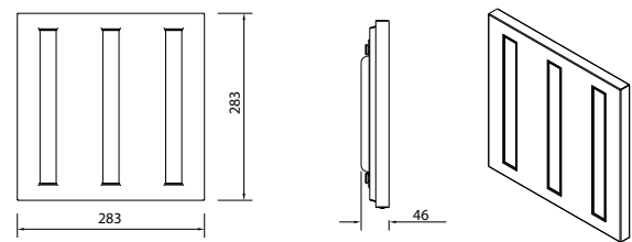
30x30 Sasled Mini Surface Mounted (3 Bar) Luminaire
